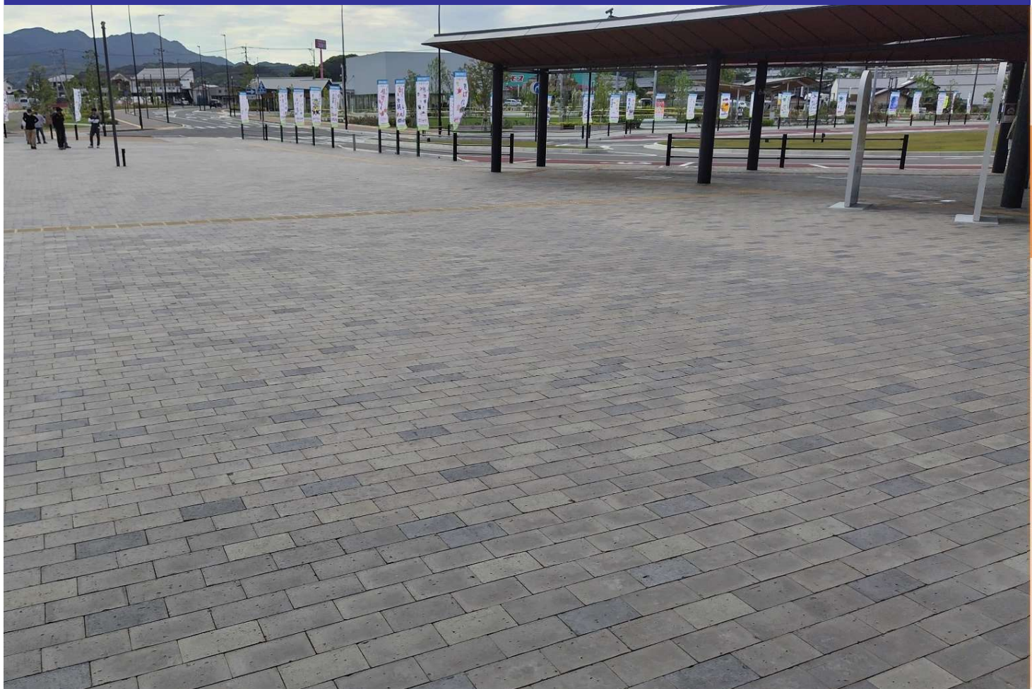
佐賀国道事務所 佐賀県嬉野市 嬉野地区簡易パーキング情報休憩施設 品名：新燃れんが 寸法：230×115×40
