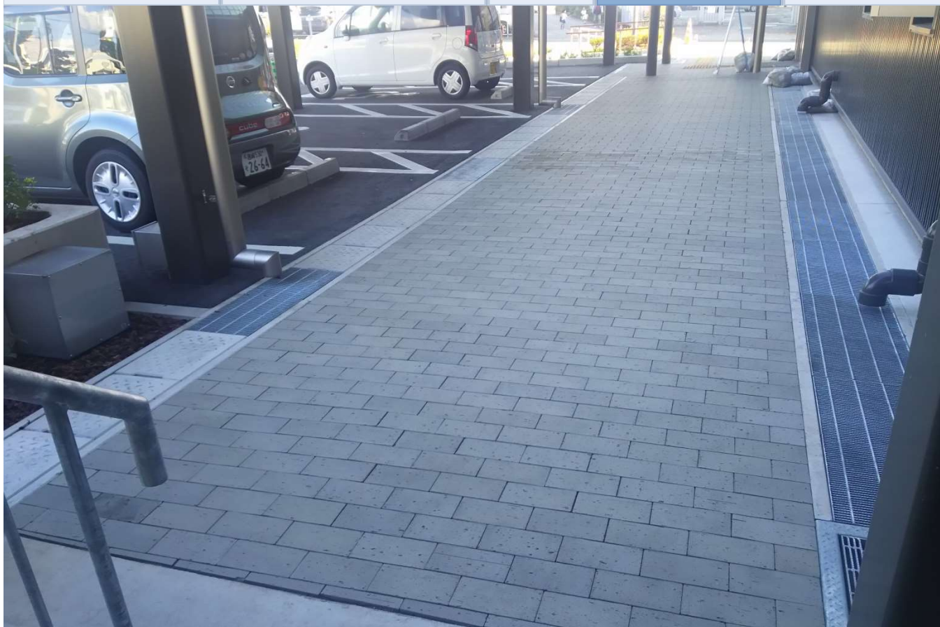
小林市役所 宮崎県小林市 小林新庁舎・外構 品名：新燃れんが 寸法：230×115×40
