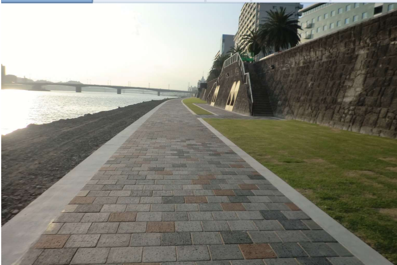
宮崎河川国道事務所 宮崎県宮崎市 大淀川 高洲地区特殊築堤 品名：新燃れんが 寸法：300×300×50
